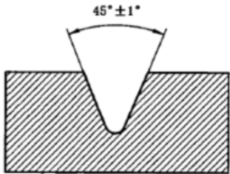
缺口底部半径 r_N = 0.25 \text{ mm} \pm 0.05 \text{ mm} a) A 型
