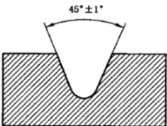
缺口底部半径 r_N = 1.00 \text{ mm} \pm 0.05 \text{ mm} b) B 型
